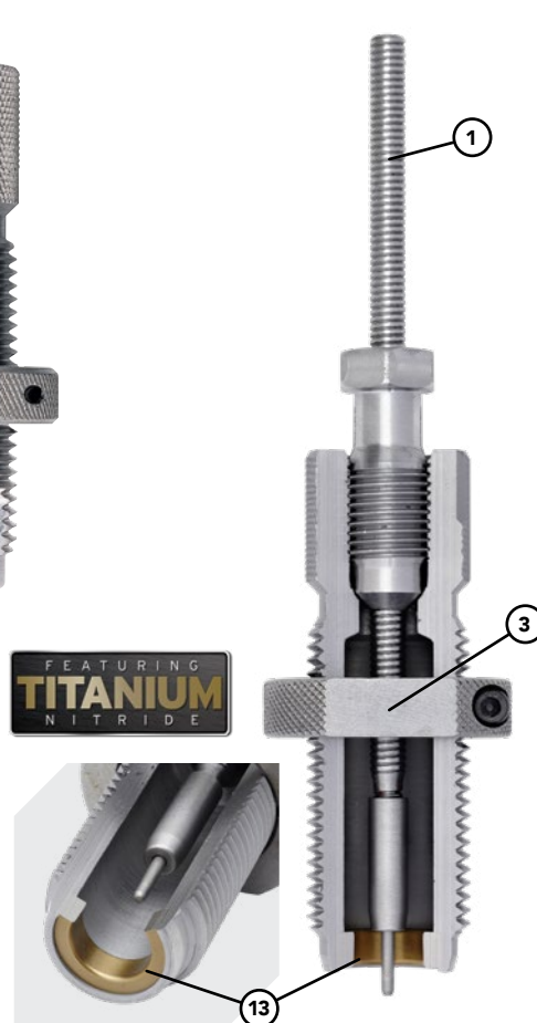
Vyměnitelný kolík (Č. 390222) je pro matrice jedinečný.
