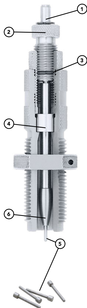
Vyměnitelný kolík (Č. 390222) je pro matrice jedinečný.
